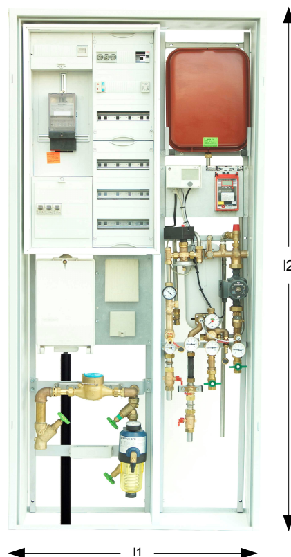
Abbildung 3: Darstellung einer Hausanschlussnische
