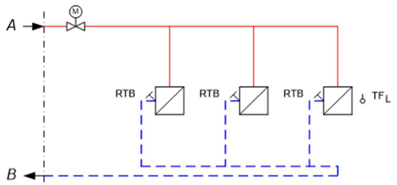
Abbildung 7: Hauszentrale-Raumluftheizung Prinzipschaltbilder für den indirekten Anschluss
