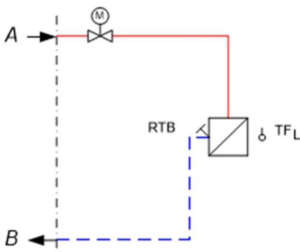
Abbildung 7: Hauszentrale-Raumluftheizung Prinzipschaltbilder für den indirekten Anschluss
