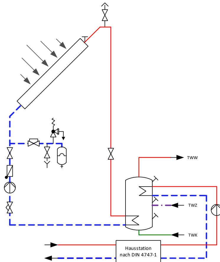
Abbildung 9: Speichersystem mit innen liegenden Heizflächen für Solar und Fernwärme
