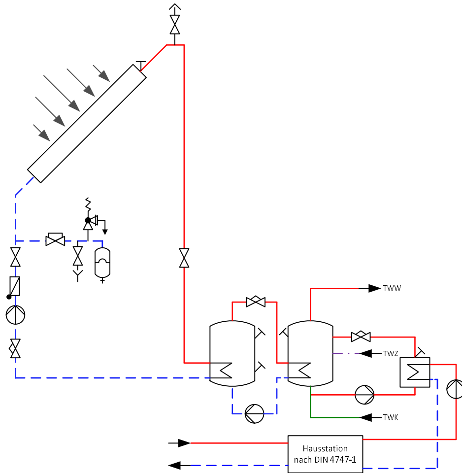
Abbildung 11: Solaranlage mit Pufferspeicher und Trinkwassererwärmer mit außen liegendem Wärmeübertrager für die Nachheizung
