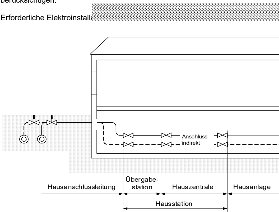
Abbildung 4: Hausanschlussleitung und Hausstation
