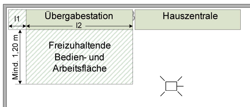
Abbildung 2: Hausanschlusswand
