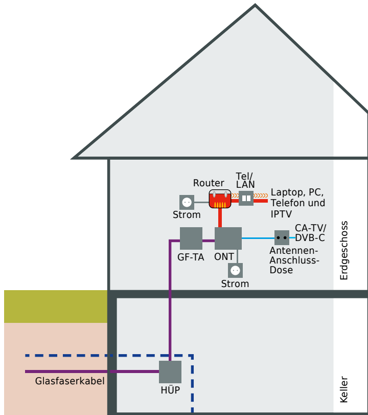
Abbildung 1: Einfamilienhaus
